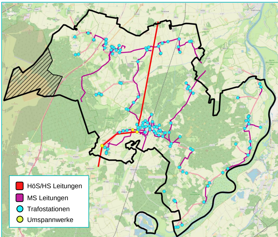
Abbildung 23: Kartografische Darstellung der IST-Wärmenetze als rote Leitungen und die entsprechenden Wärmeerzeugungsanlagen als rote Punkte (Stadt Tangerhütte – Annahme).
