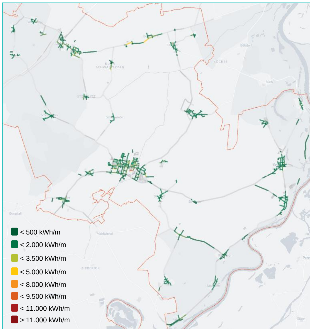
Abbildung 25: Wärmeliniendichte in kWh/m
