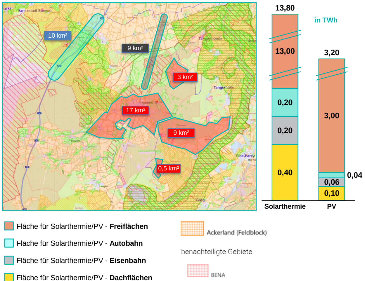
Abbildung 41: Potenzialflächen für Freiflächen-Solarthermie (links) und Potenziale bei der Nutzung aller vorhandenen Freiflächen (rechts)
