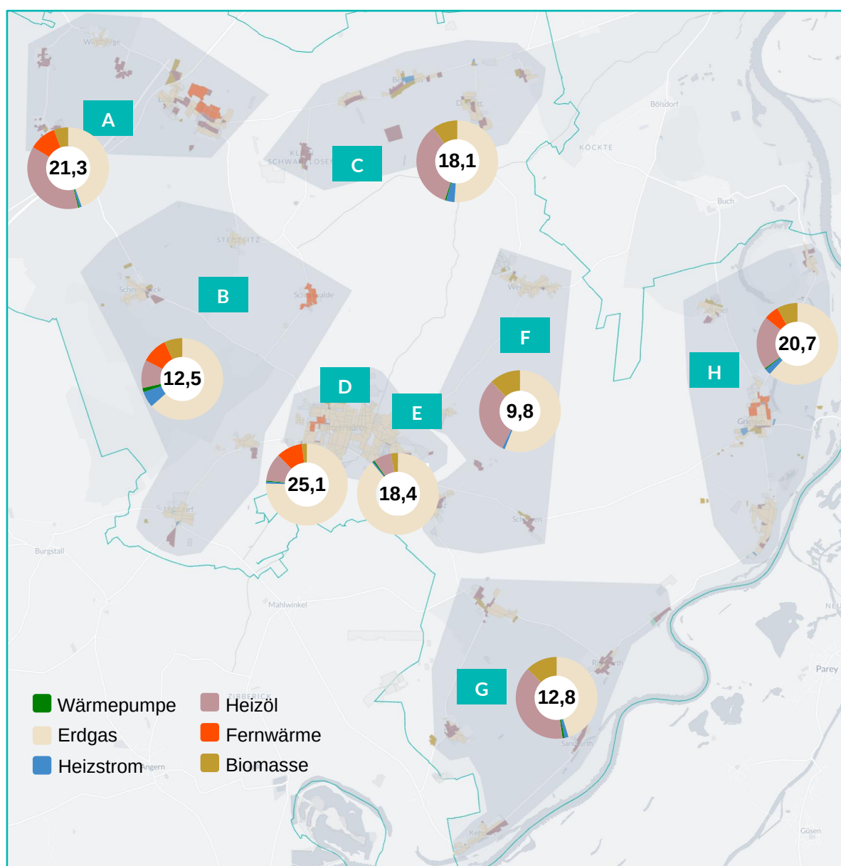
Abbildung 16: Anteil der Energieträger am jährlichen Endenergieverbrauch (in GWh/a) für Wärme in Form einer baublockbezogenen Darstellung aufgeteilt in Gebiete A bis H
