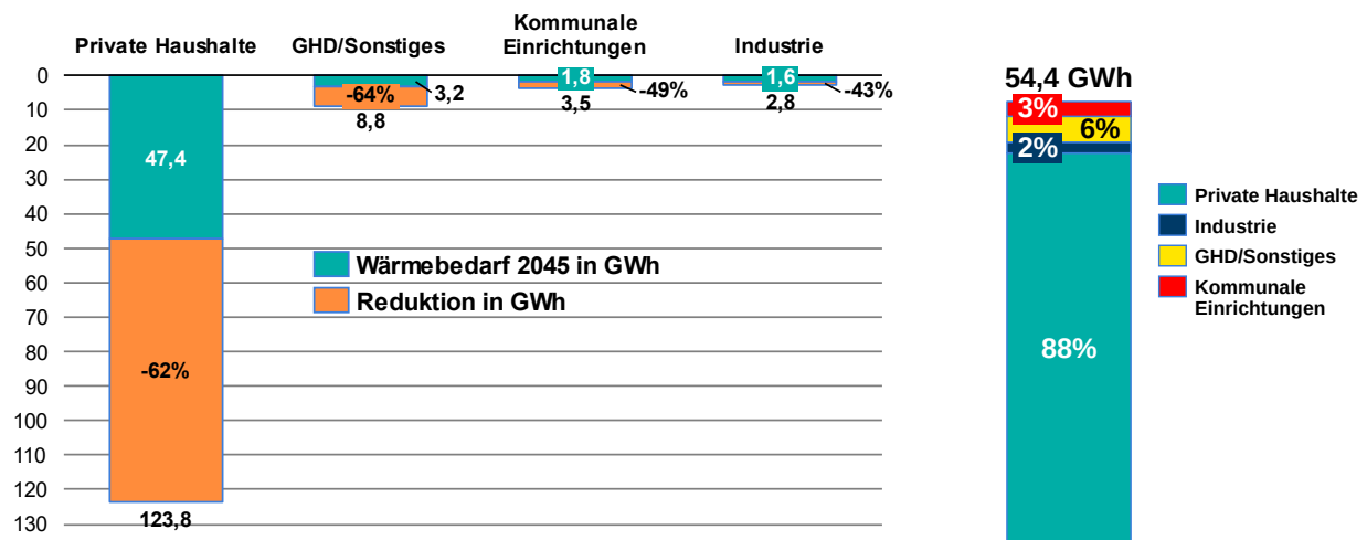
Abbildung 54: Wärmebedarf und Reduktion 2045 in GWh (links) und Anteile am Wärmeverbrauch 2045 nach BSKO-Sektoren (rechts)
