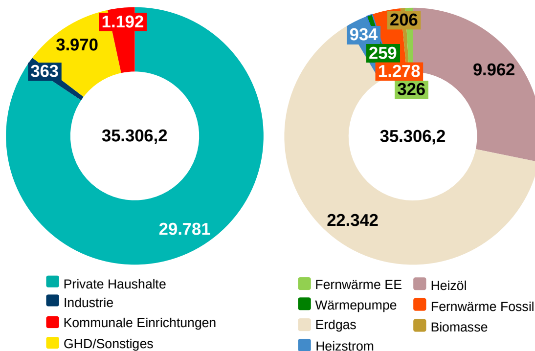
Abbildung 17: THG-Emissionen-Wärme je BSKO-Sektor (links) und Energieträger in kt/a (rechts)
