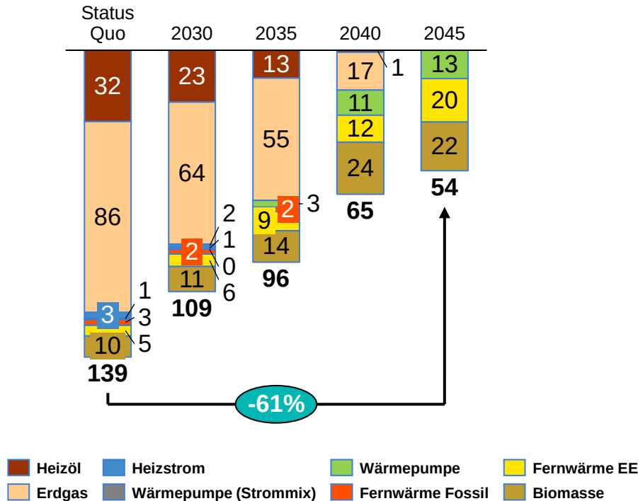
Abbildung 3: Endenergiebedarf – Wärme in GWh pro Zieljahr
