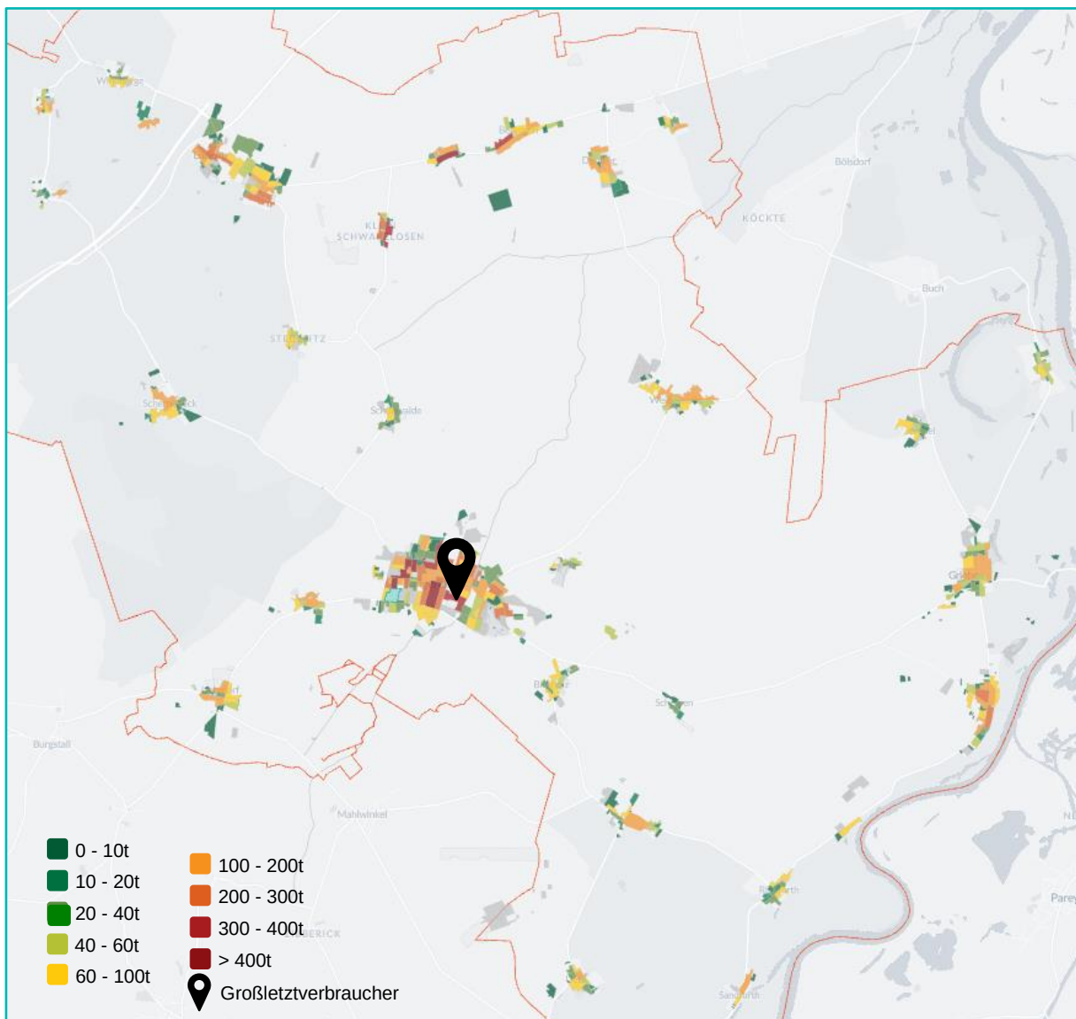
Abbildung 18: Übersicht der Wärmeemissionen (Baublockebene) und der Großletztverbraucher
