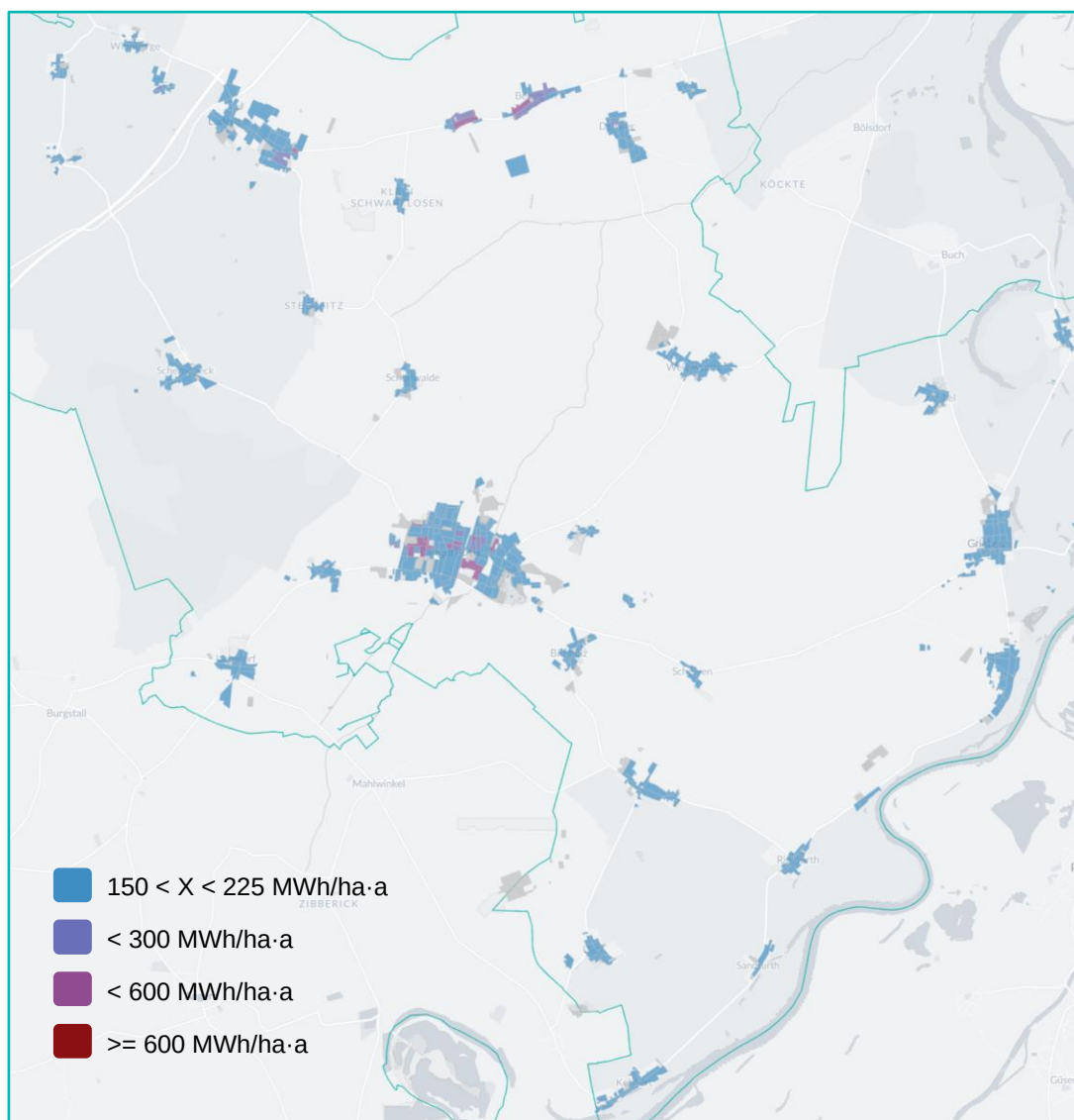
Abbildung 24: Wärmeverbrauchsichten (Endenergie) in Megawattstunden pro Hektar und Jahr (Baublock)
