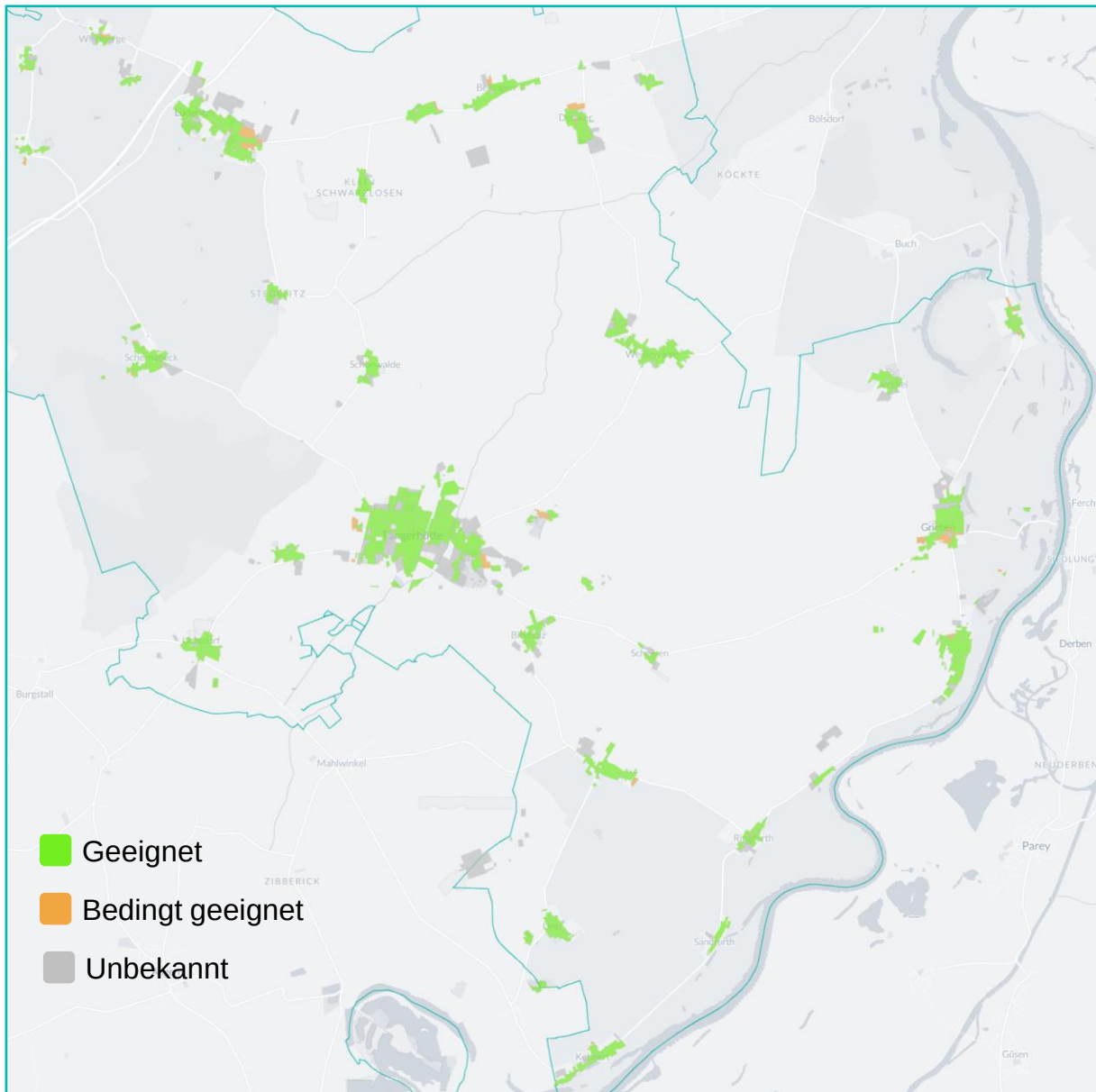
Abbildung 40: Baublockbezogene Darstellung der Wärmepumpeneignung
